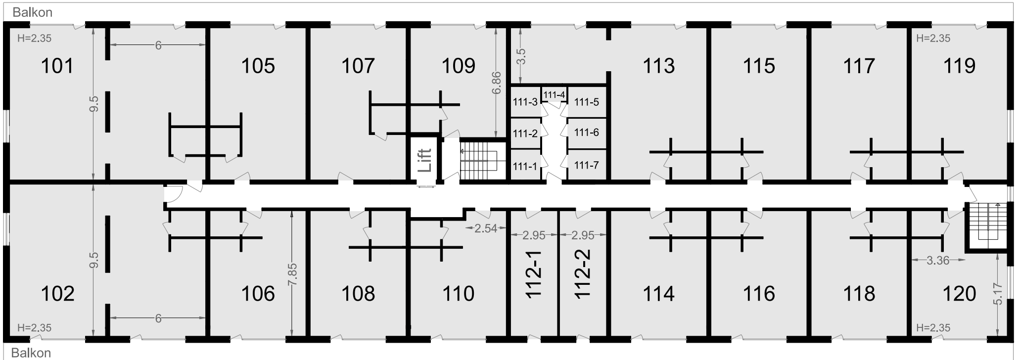
Grundrissplan 1.OG
