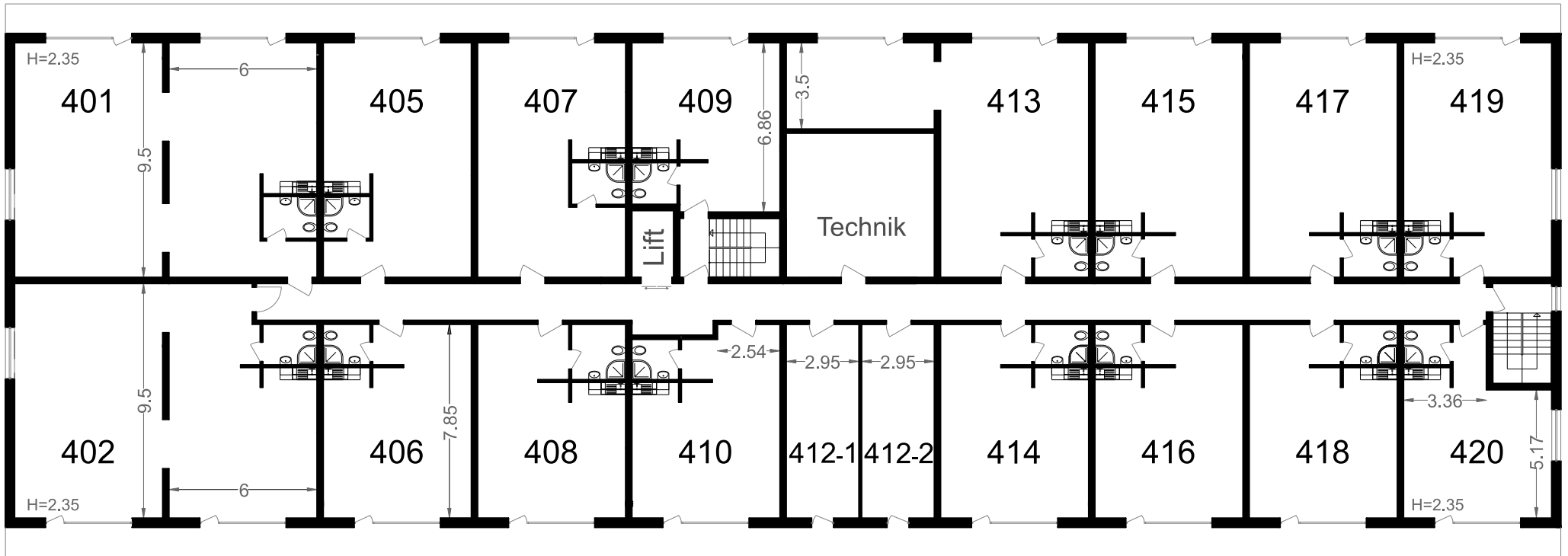
Grundrissplan 4.OG
